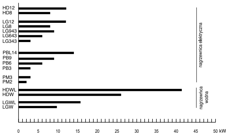
Rys. 5. Maksymalna moc grzewcza dla różnych typów kurtyk powietrznych.
