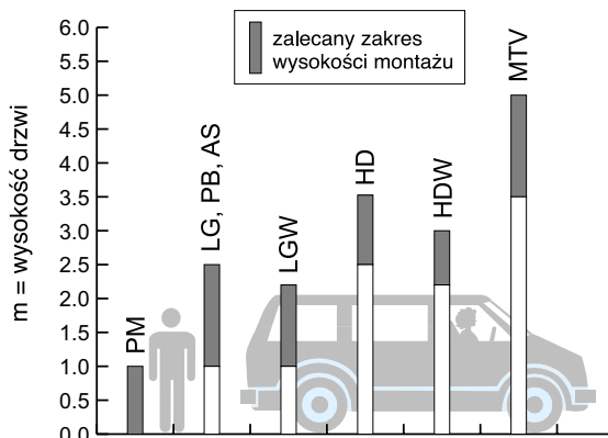
Rys. 4. Zalecane wysokości montażu kurtyk powietrznych
